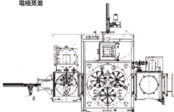
チャンパー構成例
