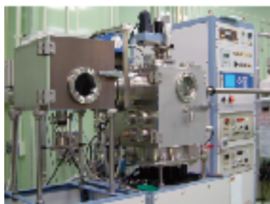
ロードロック室
